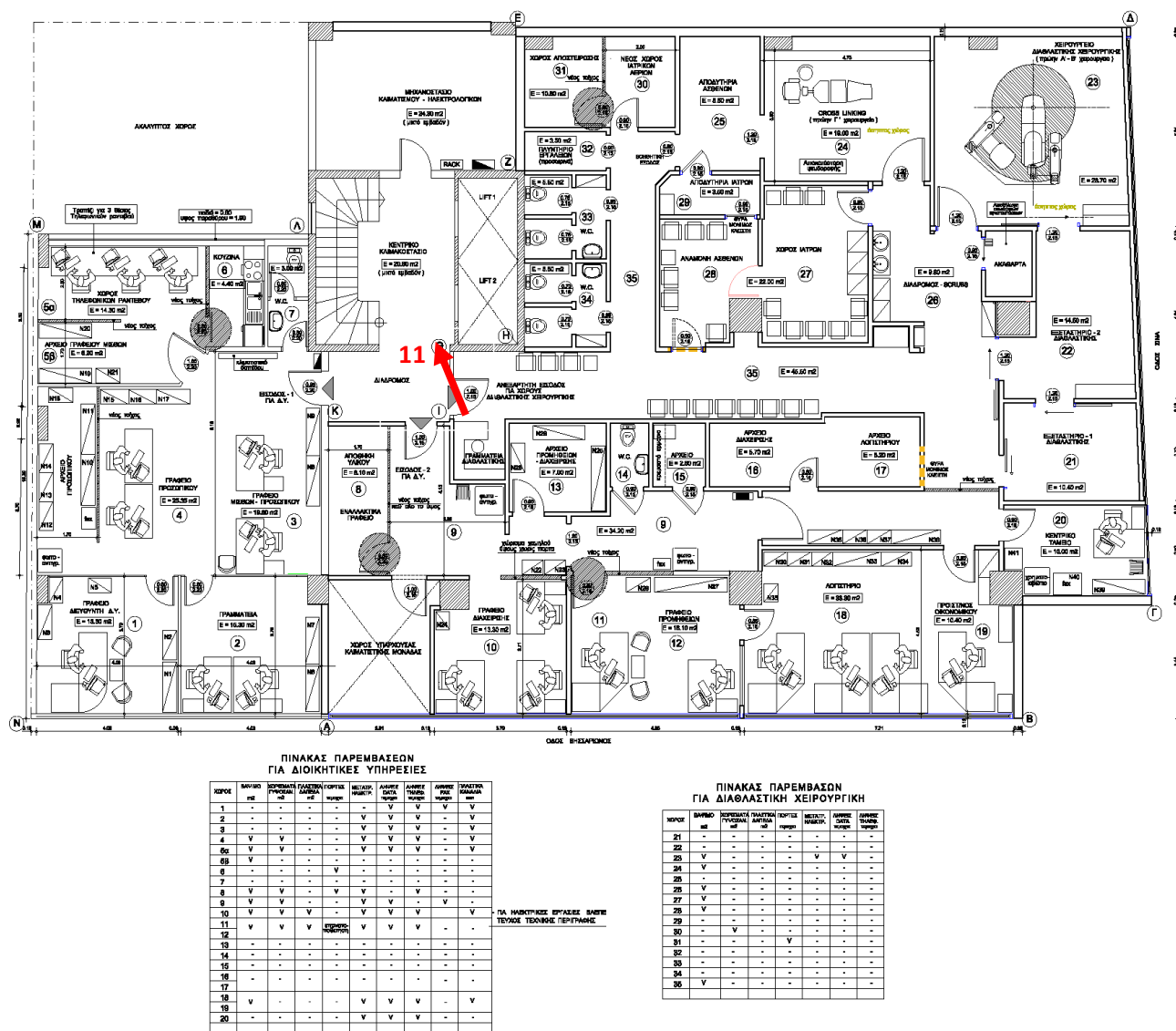
Κάτοψη 1 ου ορόφου, Βησσαρίωνος 9
