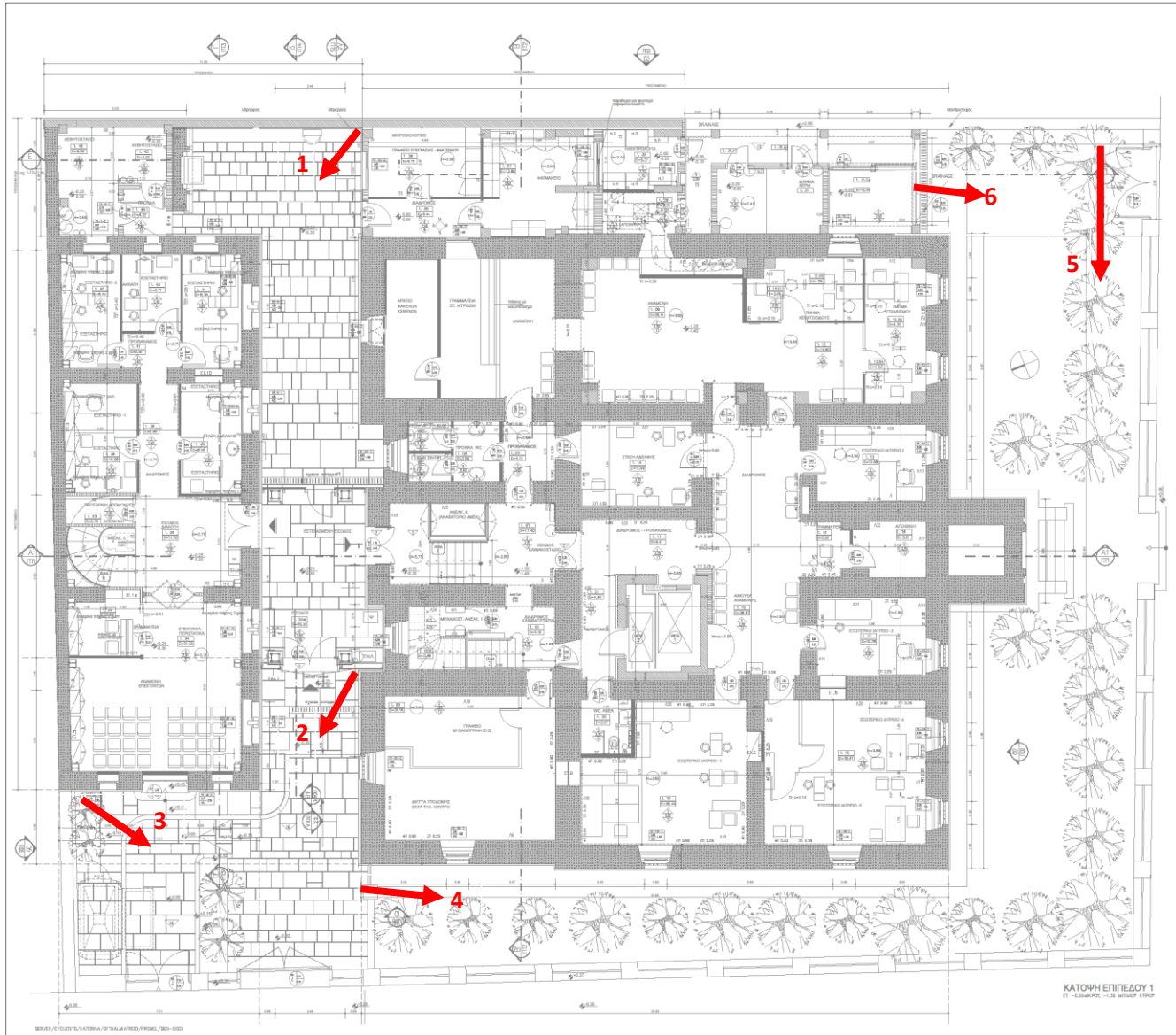
Κάτοψη Επιπέδου 1, Κεντρικό Κτήριο
