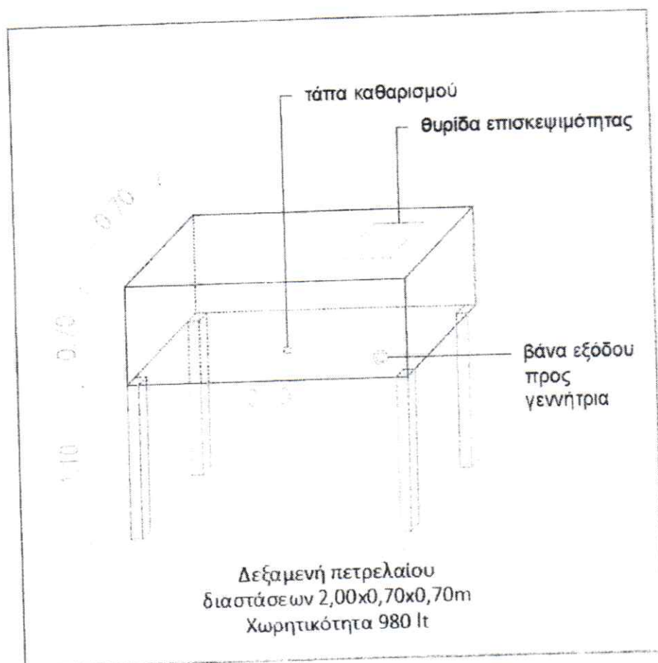
Σκαρίφημα δεξαμενής πετρελαίου
